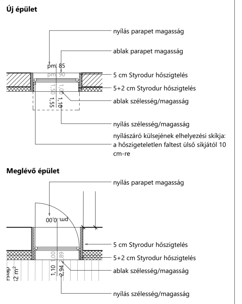
NYILÁSZÁRÓK BEÉPÍTÉSE:
